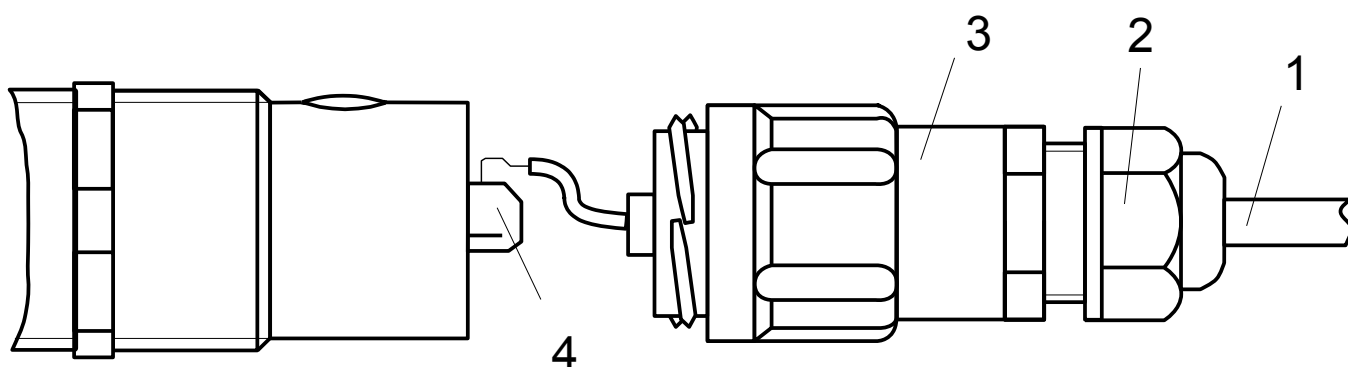
Рисунок 5 - Подключение сигнализатора
