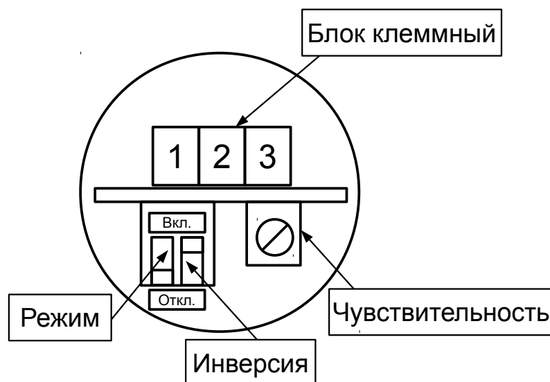
Монтажные зоны сигнализаторов исполнений СС 505.1, СС 505.2
