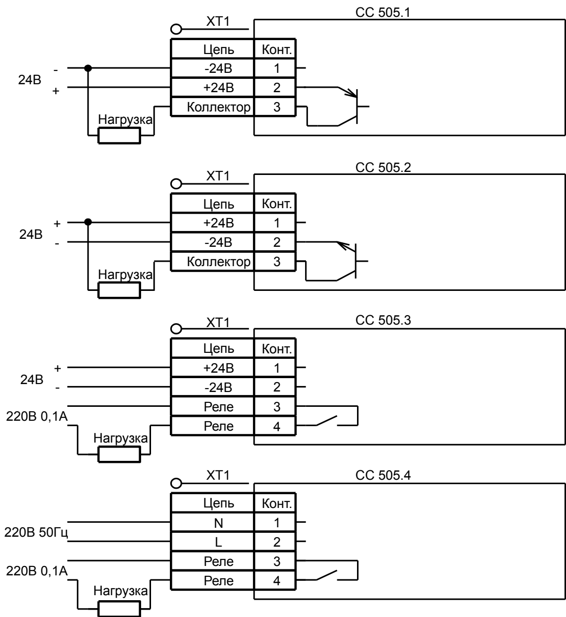
Рисунок 3 - Электрическая схема подключения
