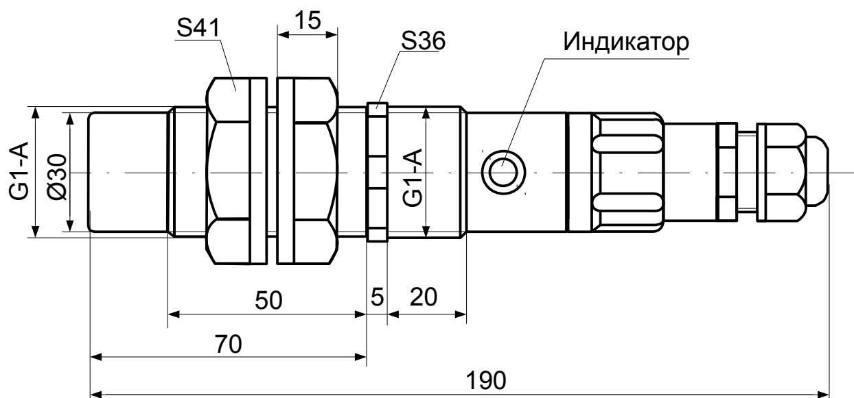
Рисунок 1 - Внешний вид и габаритные размеры
