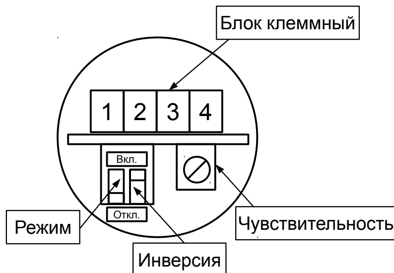
Монтажные зоны сигнализаторов исполнений СС 505.3, СС 505.4
