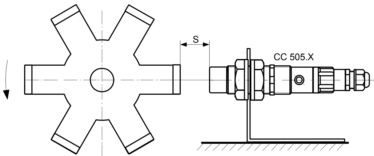
Рисунок 4 - Взаимное расположение сигнализатора и контролируемого механизма
